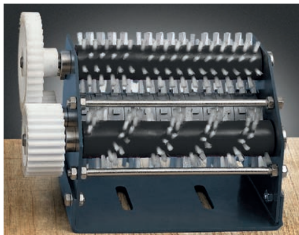
▲ Förderband-Reinigungsvorrichtung bestückt mit unseren Walzenbürsten.
